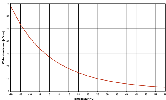
Abb. 7.1: Fühlerkennlinie NTC 10
