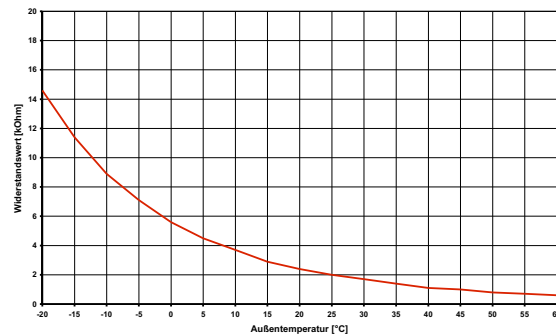
Abb. 7.2: Fühlerkennlinie NTC-2 nach DIN 44574 Außentemperaturfühler
