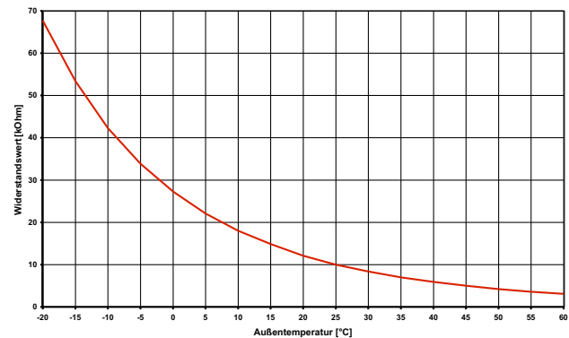
Abb. 7.2: Fühlerkennlinie NTC-10
