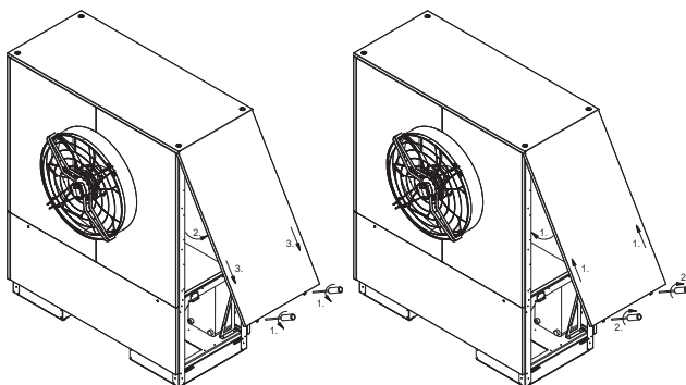
Ouverture des tôles de couvercle de côté et arrière, vue de haut Fermeture des tôles de couvercle de côté et arrière, vue de haut
