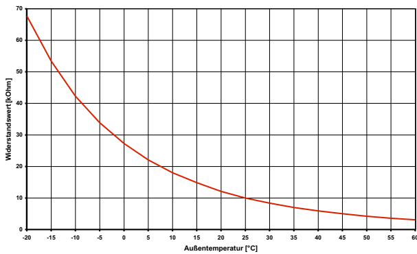
Abb. 7.1:Fühlerkennlinie NTC-10
