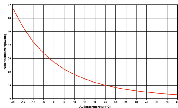
Abb. 7.2: Fühlerkennlinie NTC-10
