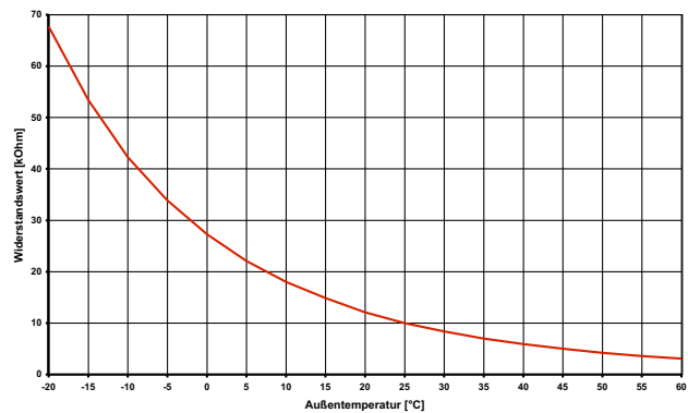
Abb. 7.2: Fühlerkennlinie NTC-10
